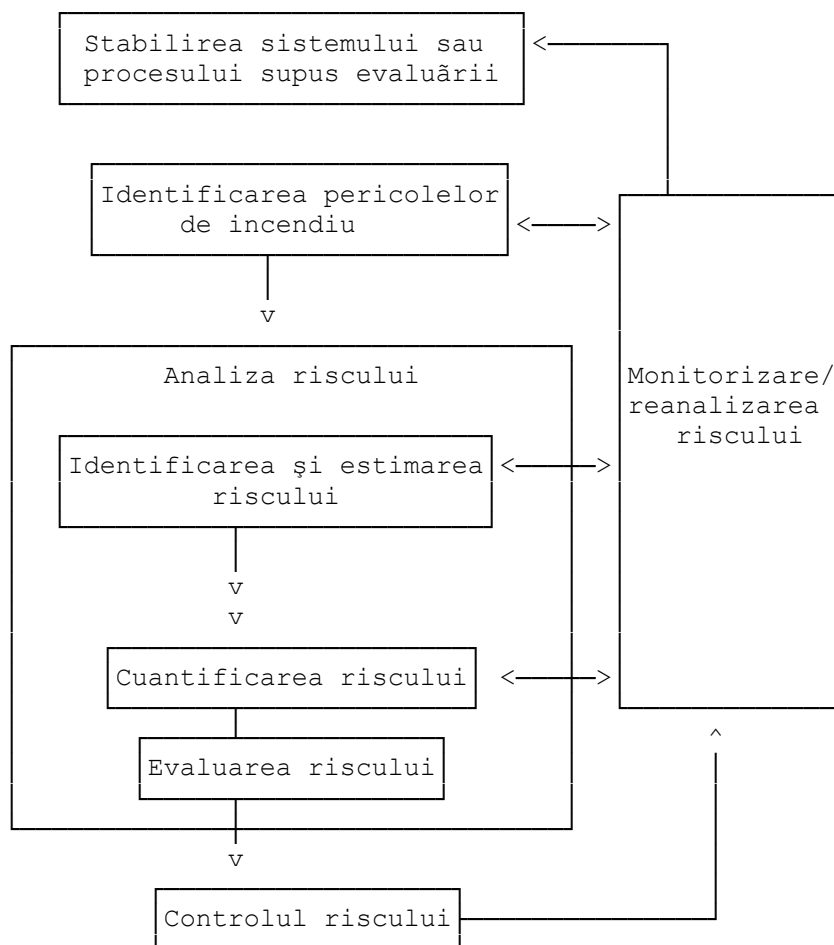
Schema logica de management al riscurilor de incendiu în faza de exploatare
