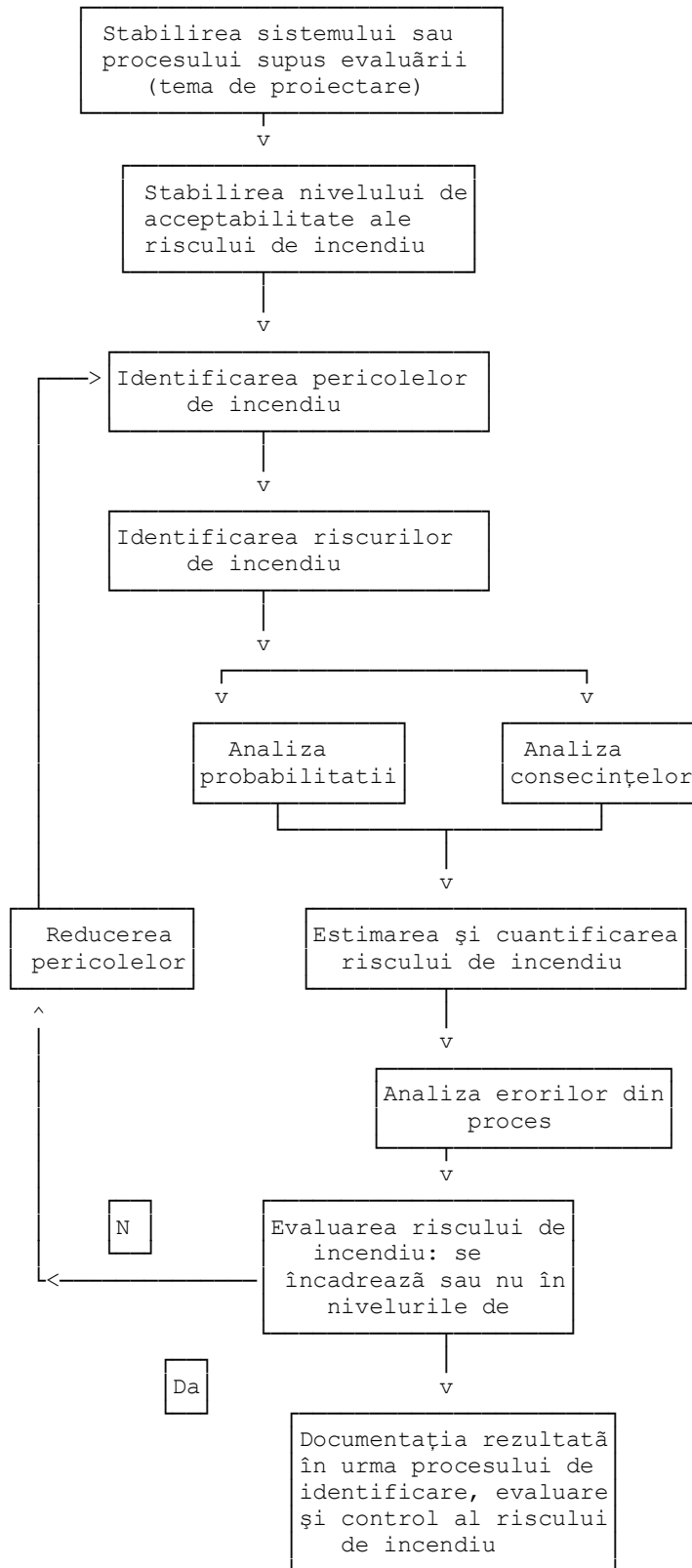
Schema logica de management al riscurilor de incendiu în faza de proiectare
